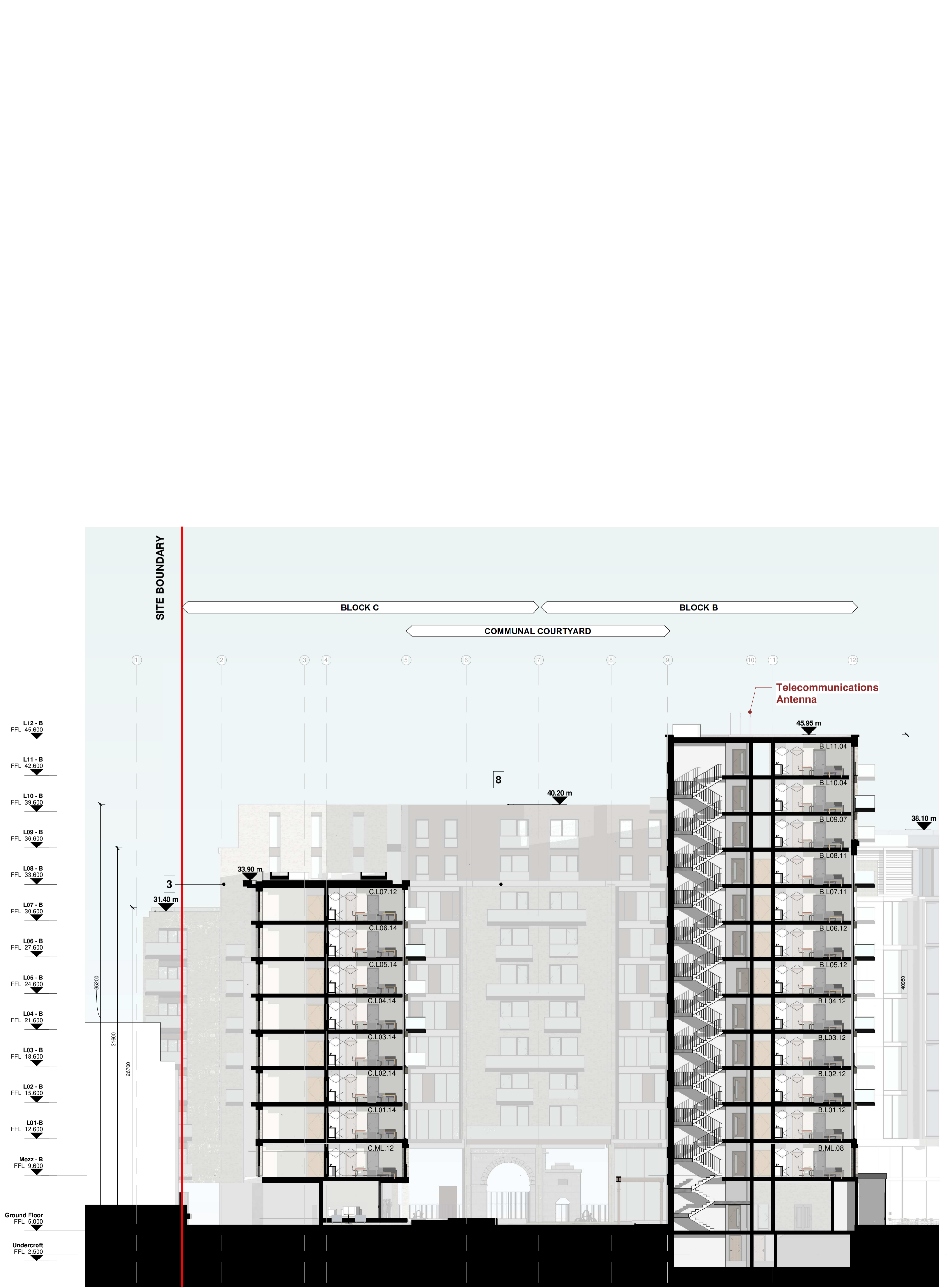
Section 1 - 1 1 : 200
