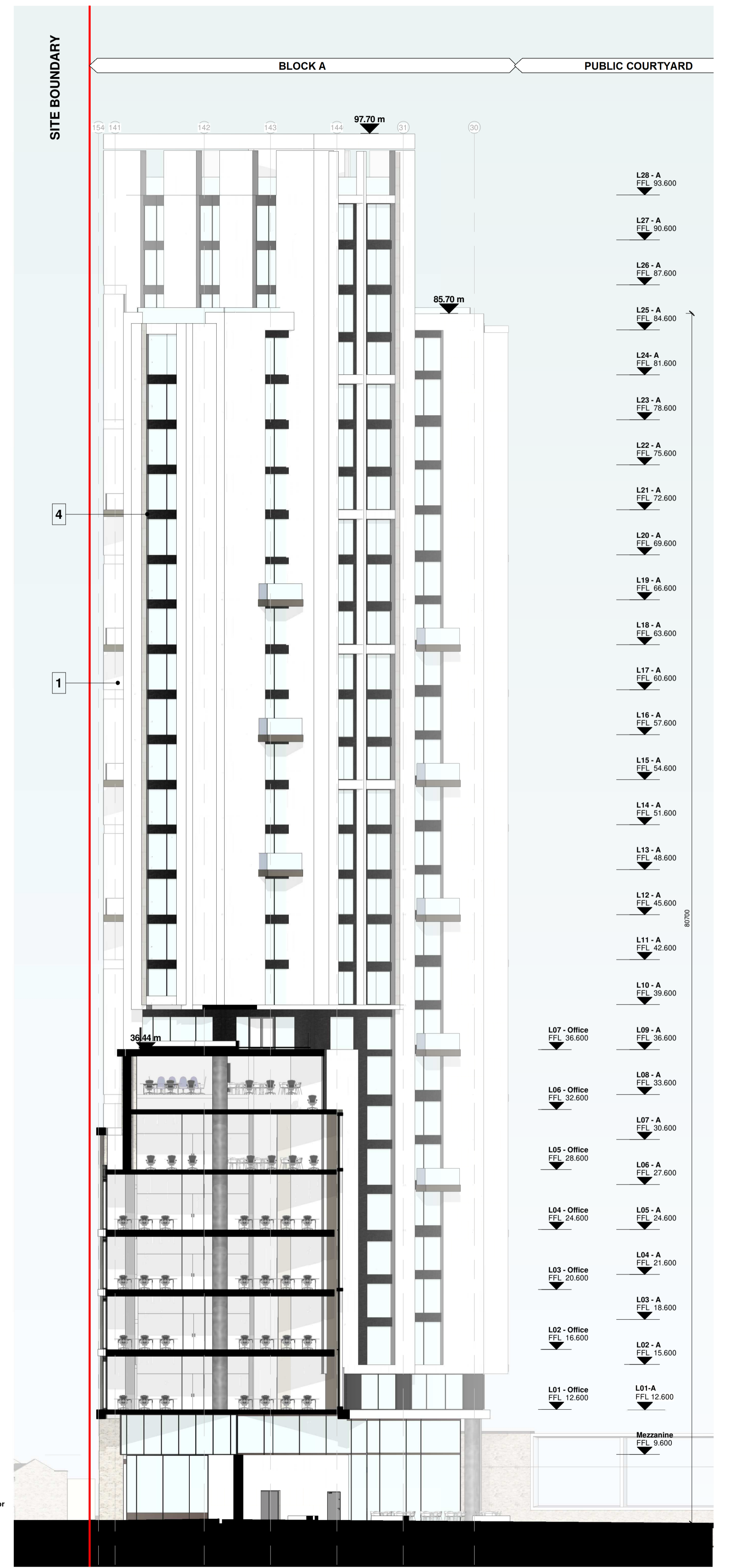
Section 2-2 1 : 200
